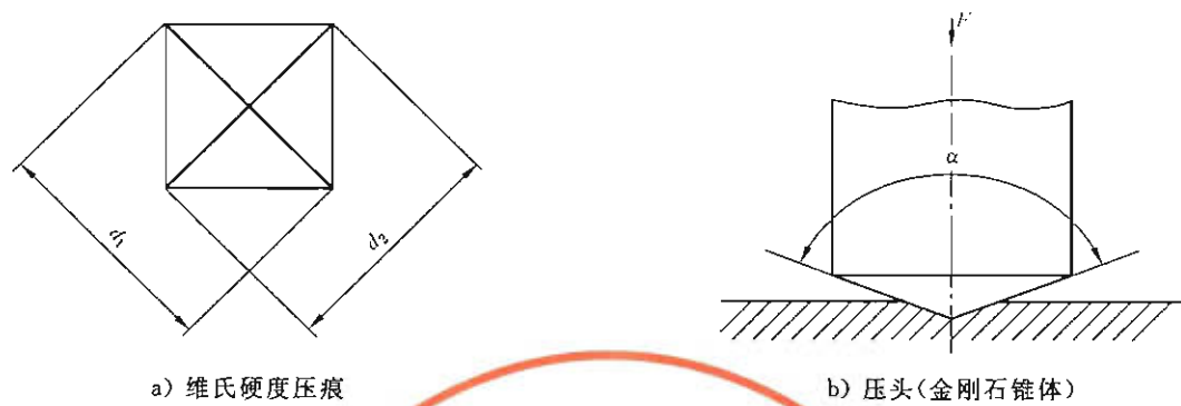
图 1 试验原理
