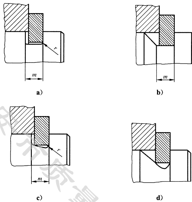
图 6 沟槽形状
