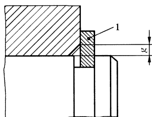
图 3 直角接触
