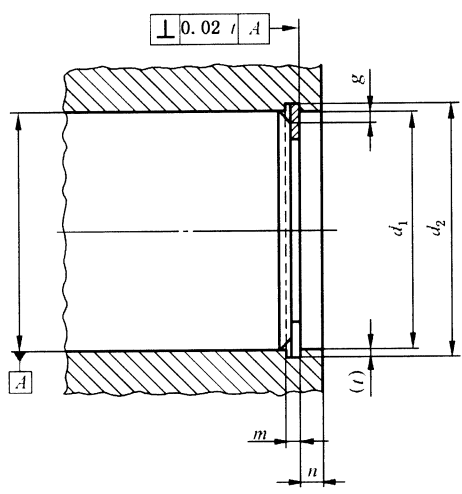
图 2 安装示例
