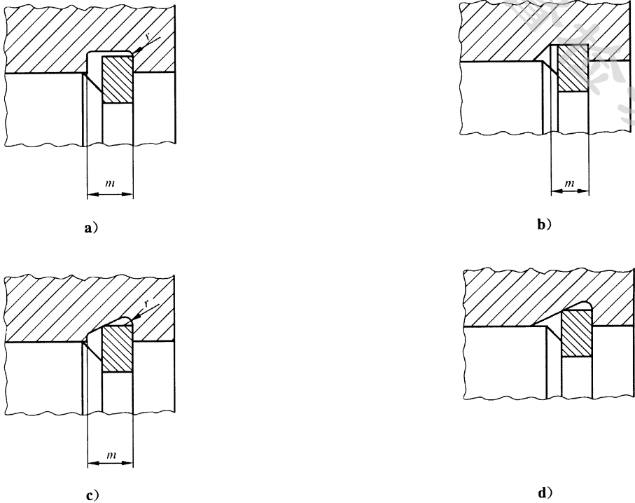
图 6 沟槽形状
