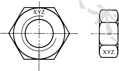
图 4 标志代号示例
