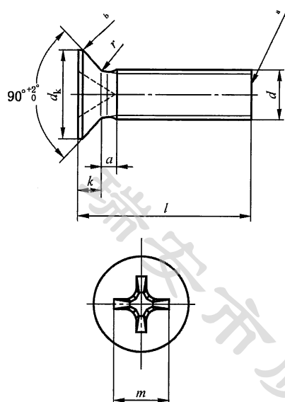
a) H 型十字槽
