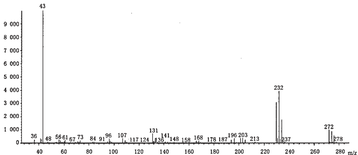
图 D.1 2,3,5,6-四氯苯酚乙酸酯标准物的气相色谱-质谱图
