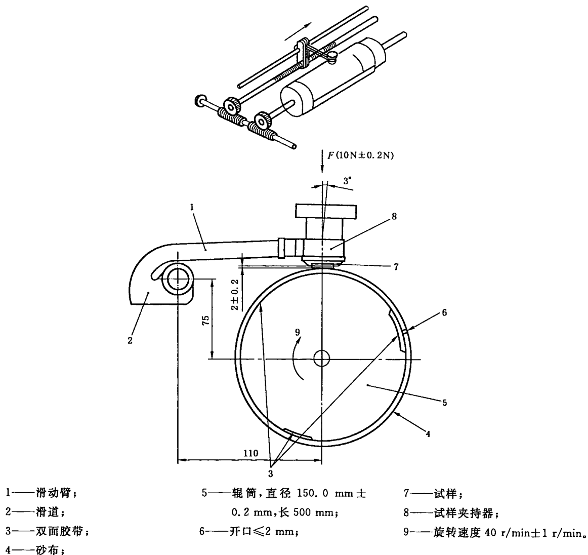
图 1 仪器结构原理图
