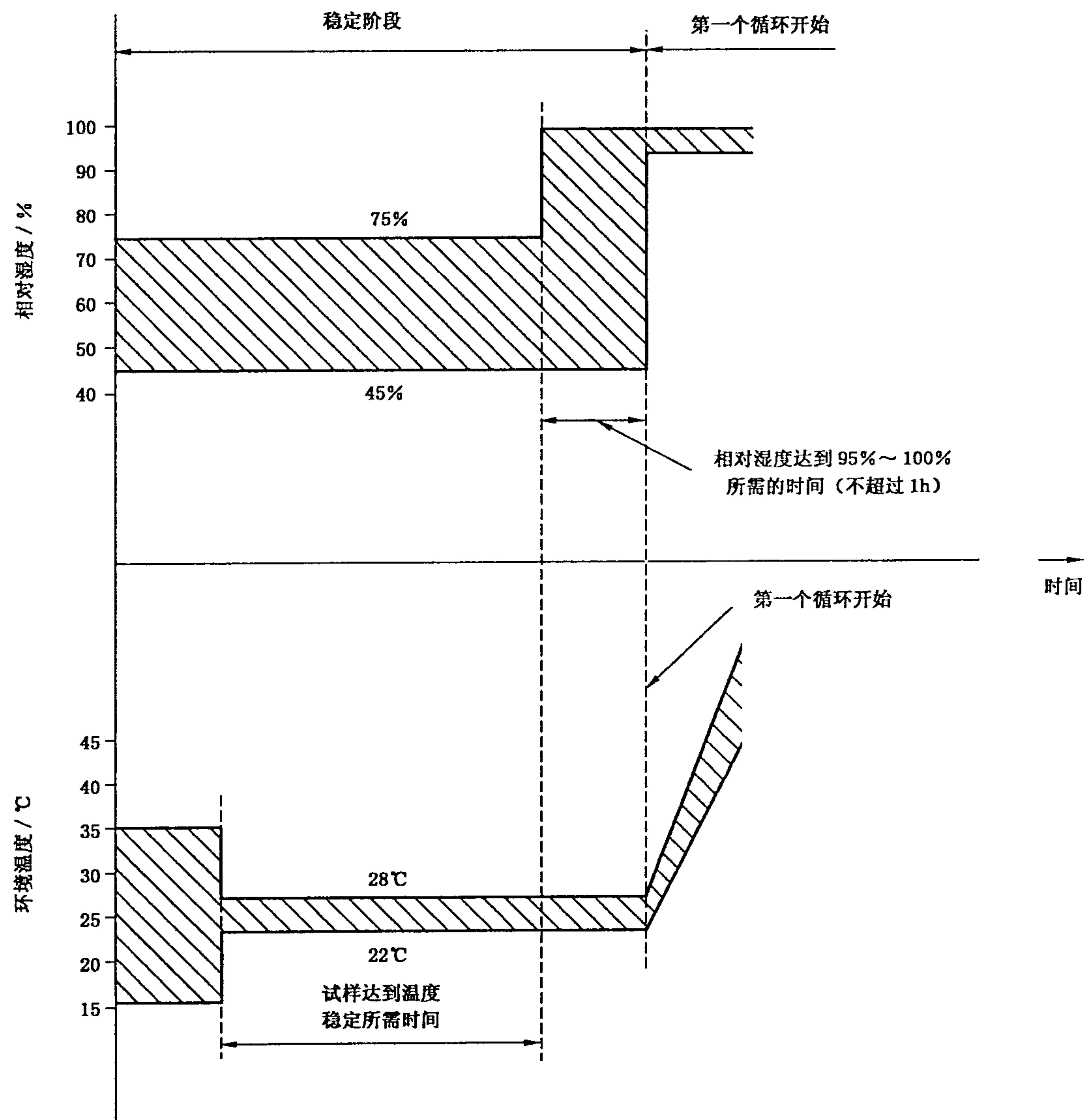
图 1 试验 Db——稳定阶段
