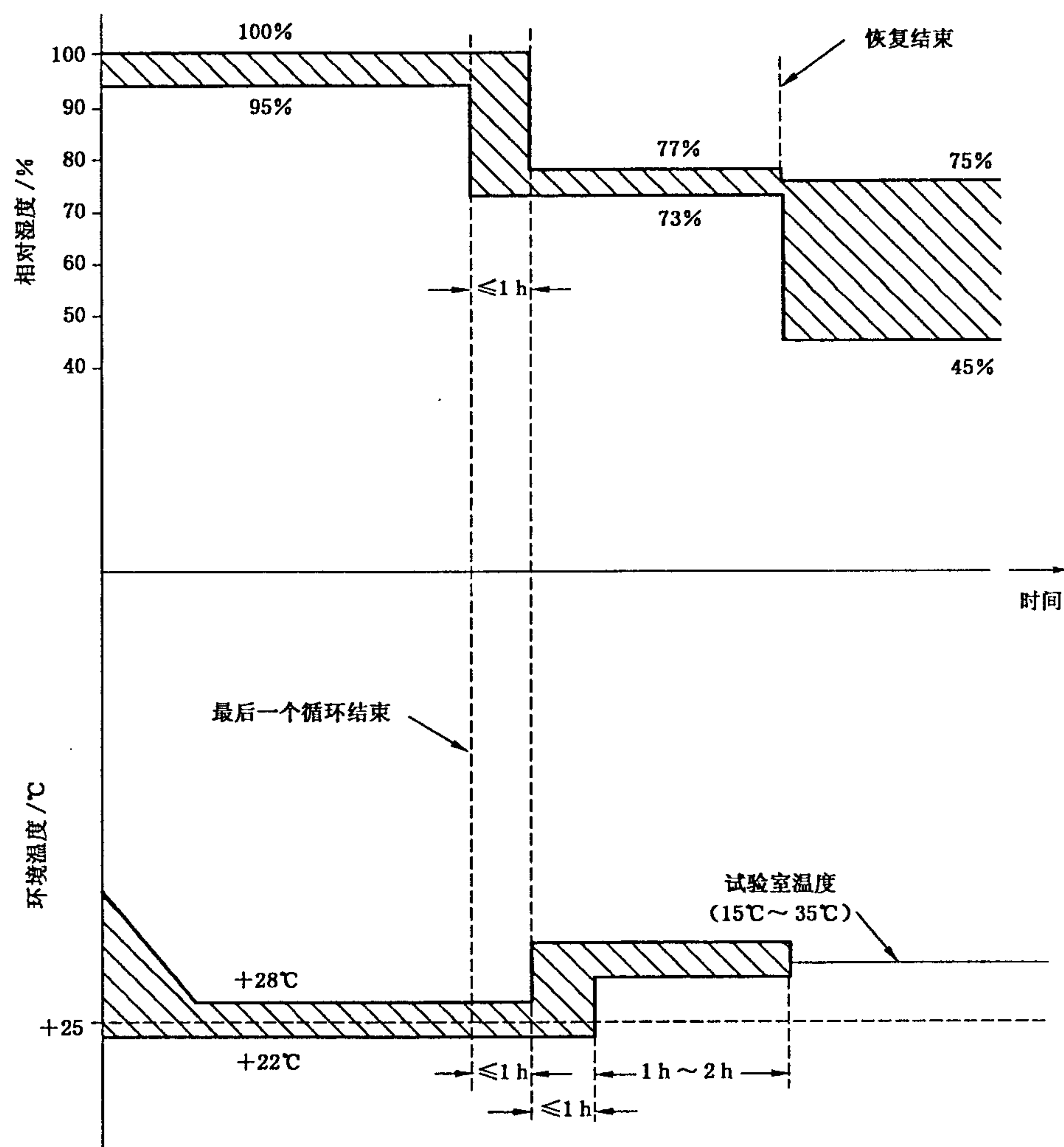
图 3 试验 Db——受控条件下的恢复
