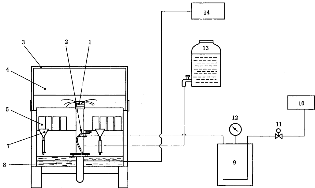
附录 A (资料性附录) 盐雾箱设计简图
