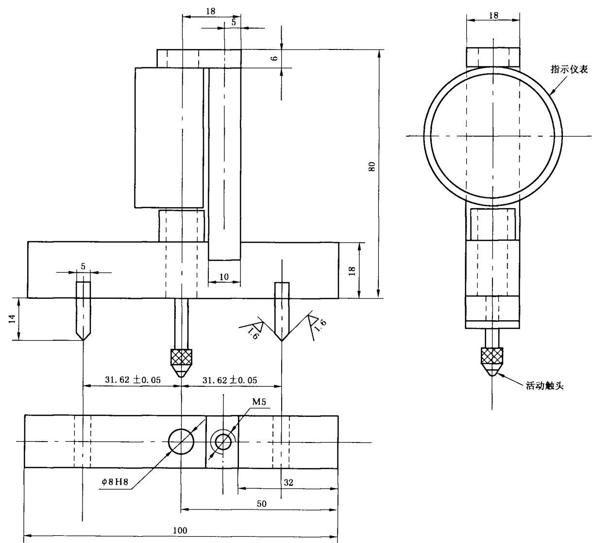
图 C.1 球面计示意图
