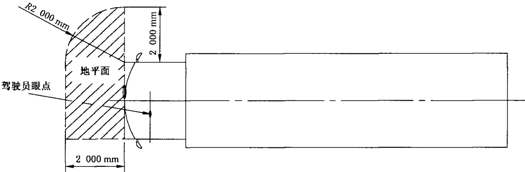
图 9 VI类前视镜的视野
