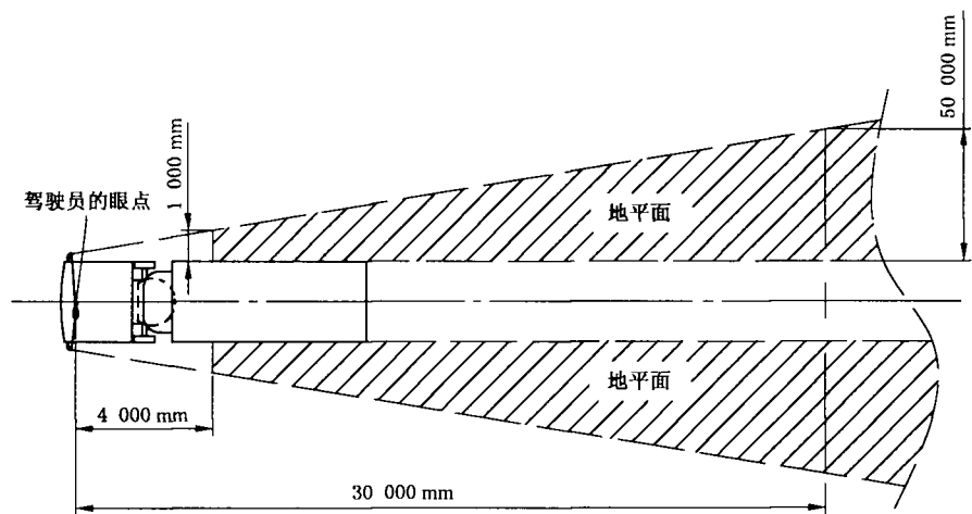
图 5 II类主外视镜的视野
