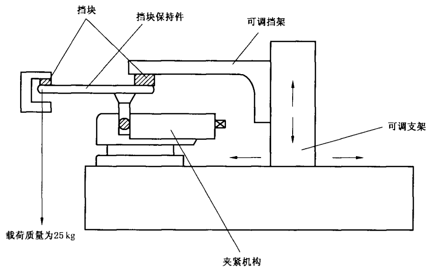
图3 视镜保护壳体弯曲试验设备示例
