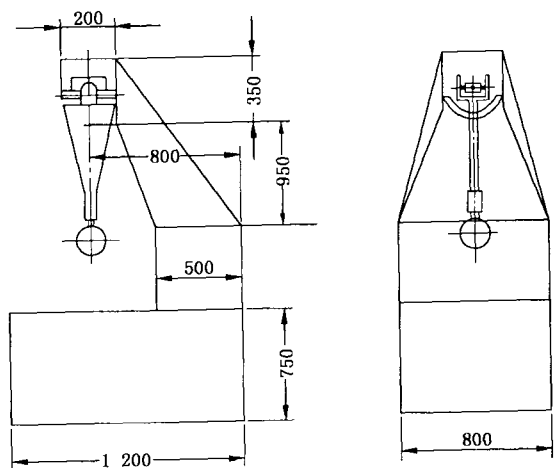
图 2 撞击试验设备示例
