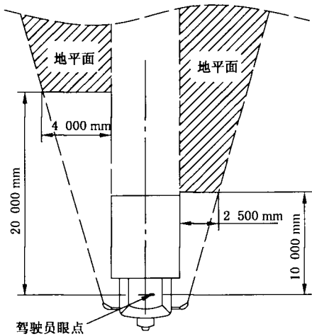
图 10 VII类视镜视野
