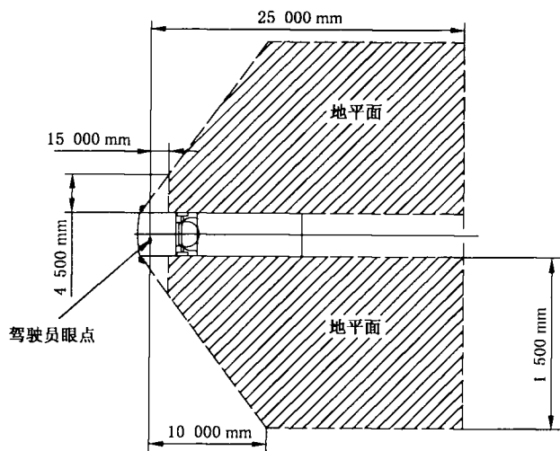
图 7 IV类广角外视镜的视野
