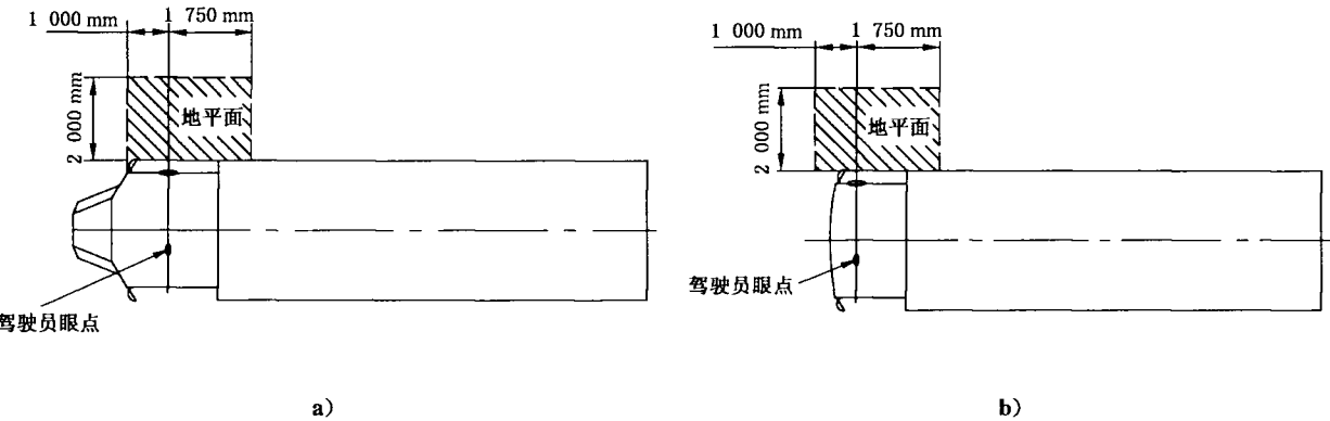
图 8 V类补盲外视镜的视野
