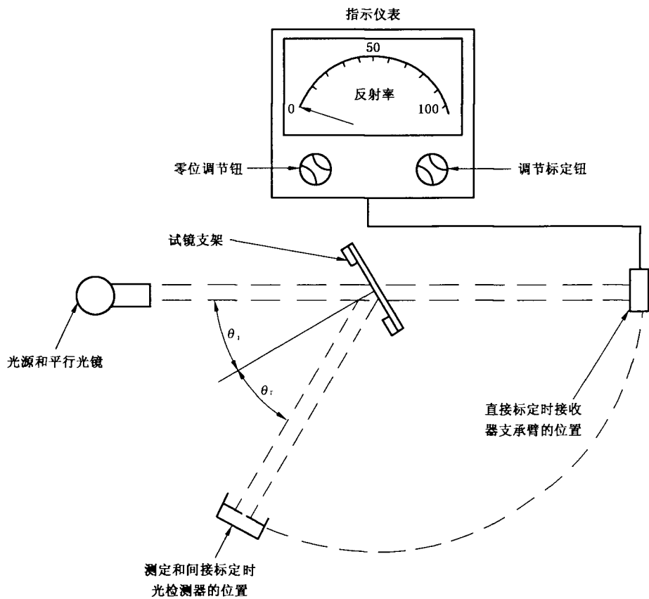
图 B.1 两种标定方法所用反射率测定仪的几何关系
