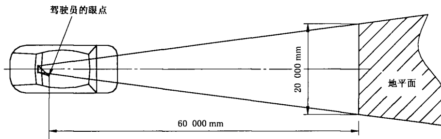
图 4 Ⅰ类内视镜视野
