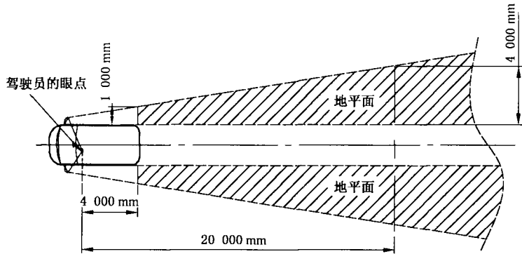
图 6 III类主外视镜的视野
