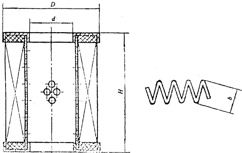
D—滤芯端盖外径；d—滤芯端盖孔径；H—滤芯高度；b—滤纸折宽
