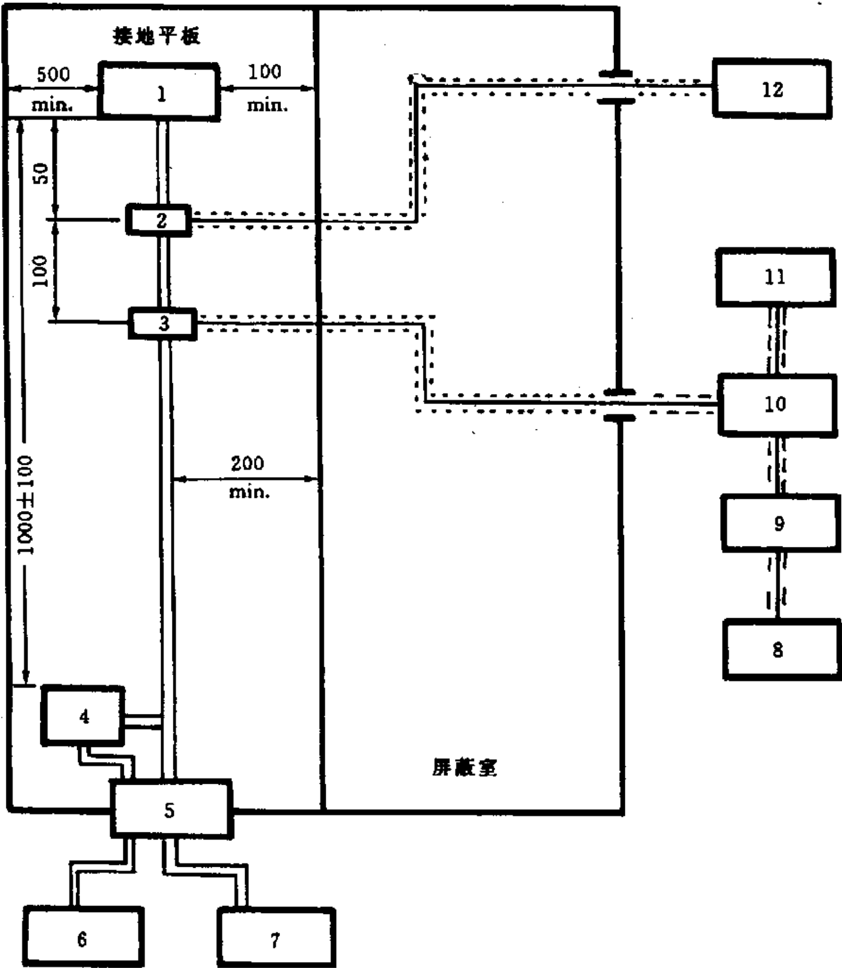
1—被测 ESA; 2—RF 测量探头(选用); 3—RF 注入探头; 4—人工网络; 5—屏蔽室滤波网络 6—电源; 7—被测 ESA 接口模拟和监视设备; 8—信号发生器; 9—宽带放大器; 10—RF 50Ω 定向耦合器; 11—RF 功率电平测试设备或等效设备; 12—频谱分析仪或等效设备(选用)
