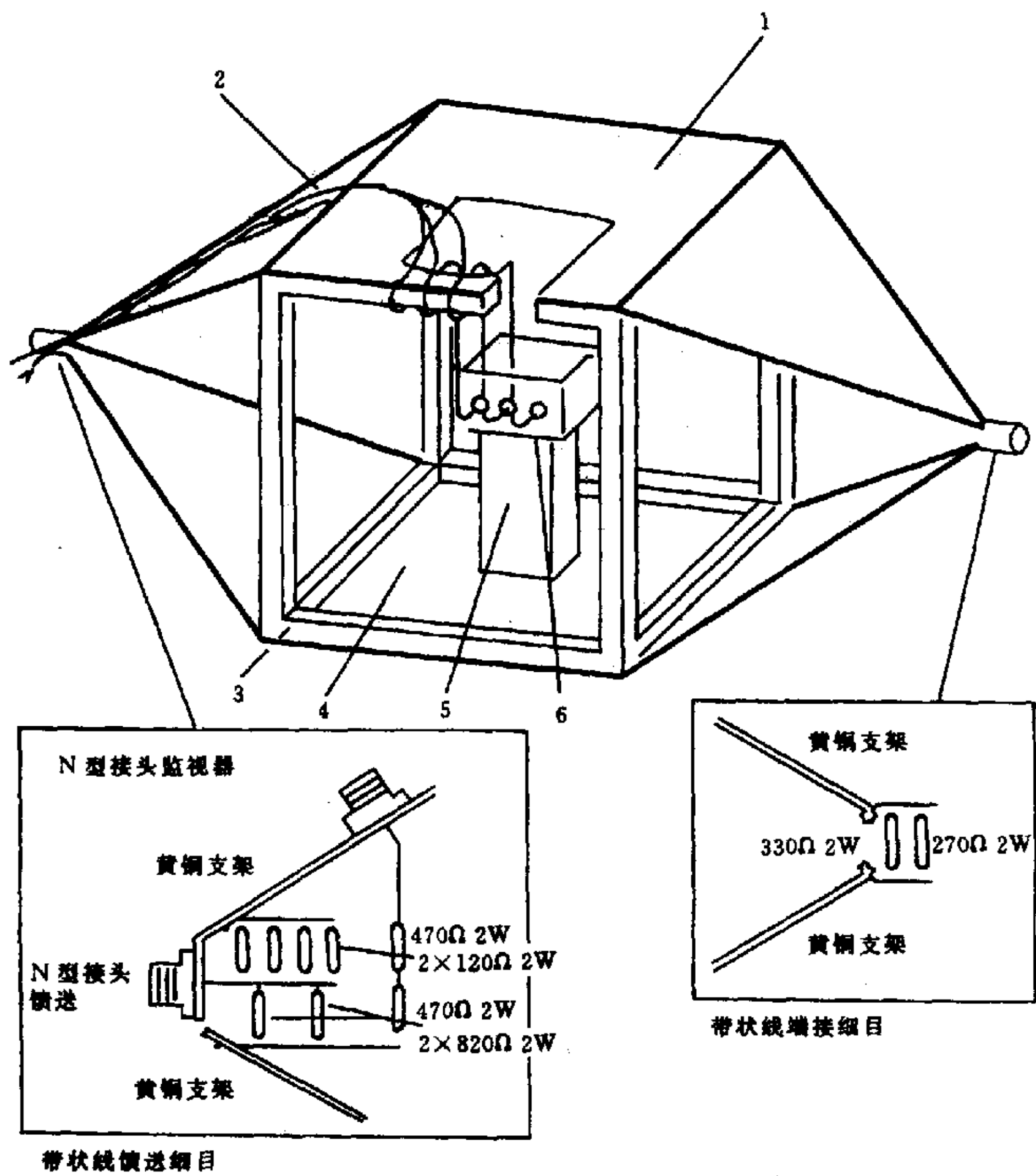
1—接地平板;2—主保护套和传感器电缆或激励器电缆;3—木质框架; 4—激励板;5—绝缘装置;6—被测物体
