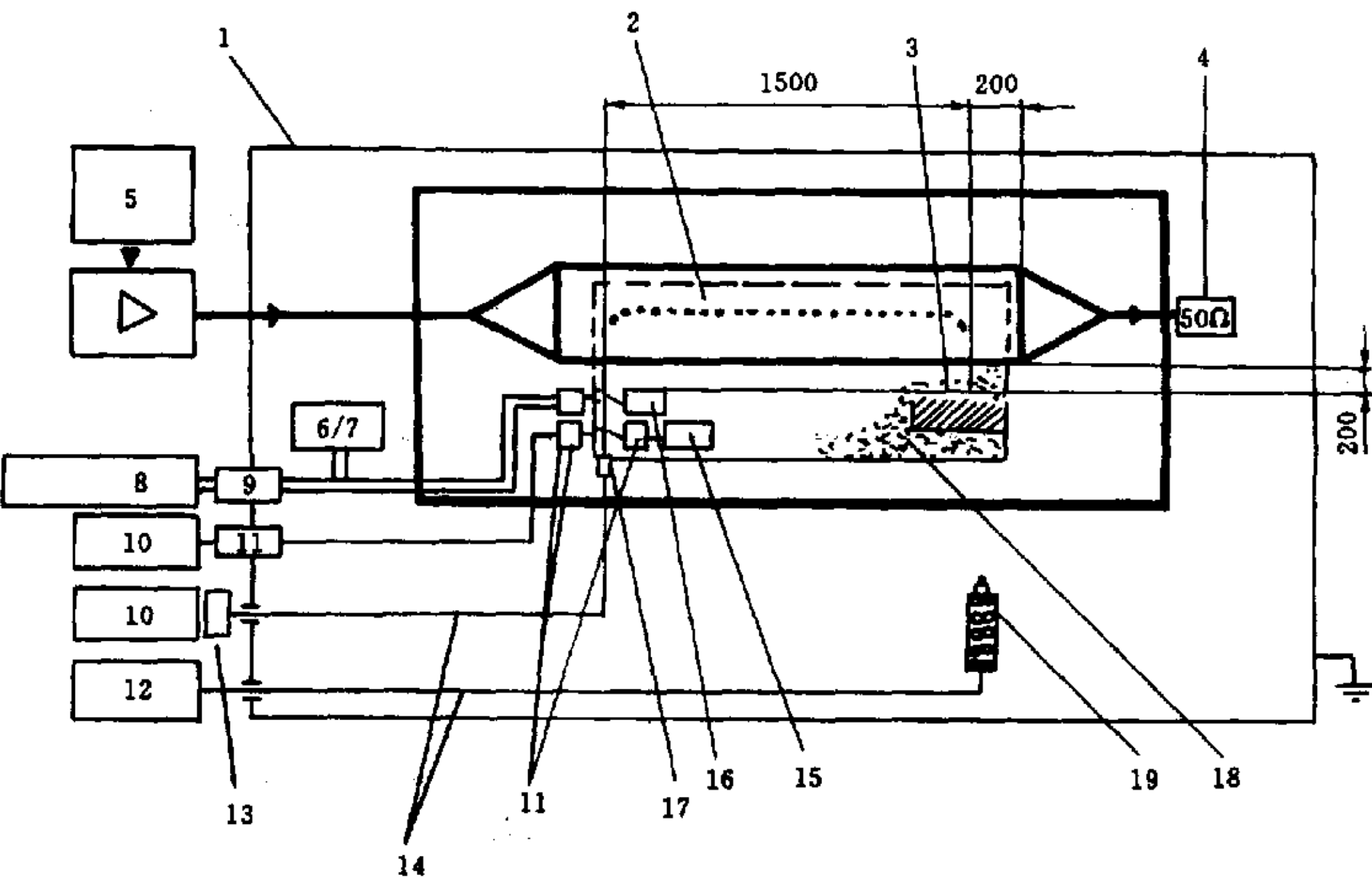
1—屏蔽室；2—电缆线束；3—被测物体；4—端接电阻；5—信号发生器；6/7—可替换的电瓶；8—电源； 9—滤波器；10—外部设备；11—滤波器；12—视频监视器；13—光电转换器；14—光缆；15—无防辐射的外设； 16—线性或防辐射外设；17—光电转换器；18—绝缘支承座；19—摄像机
