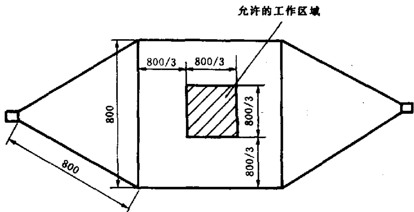
平面图
