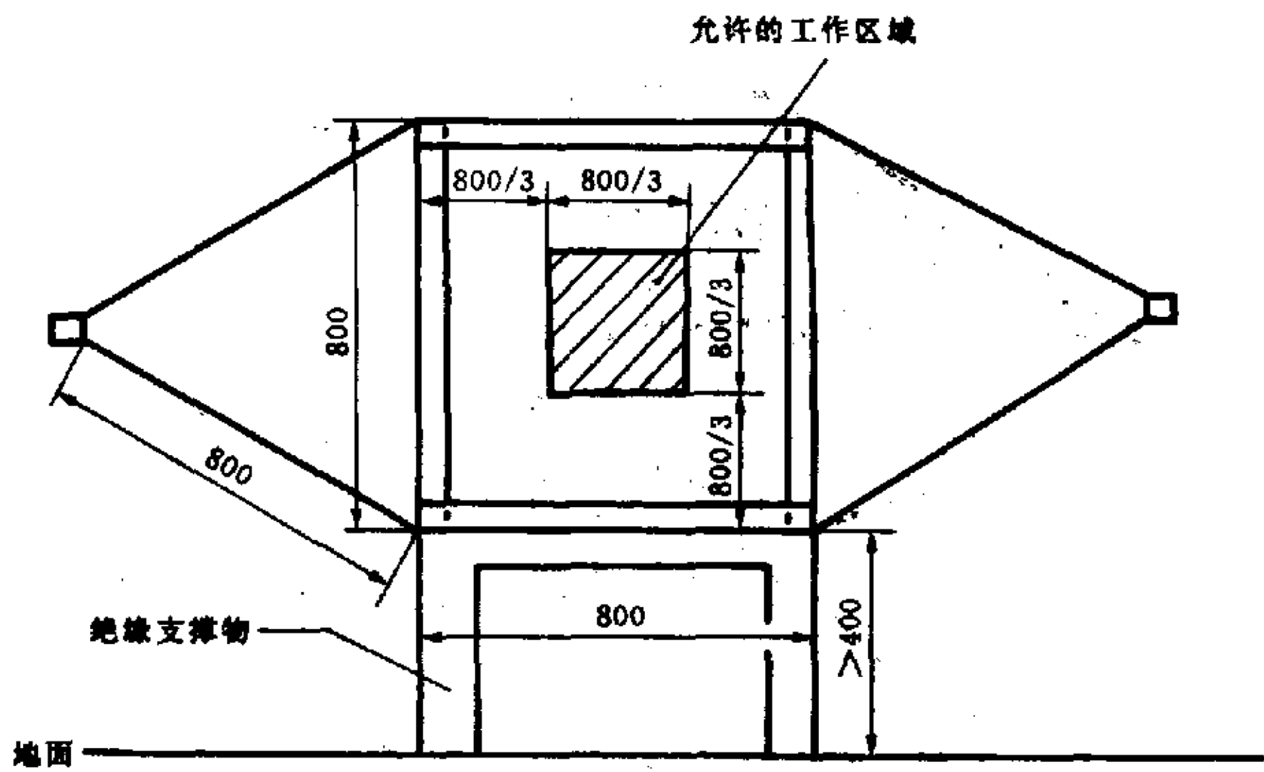
侧视图
