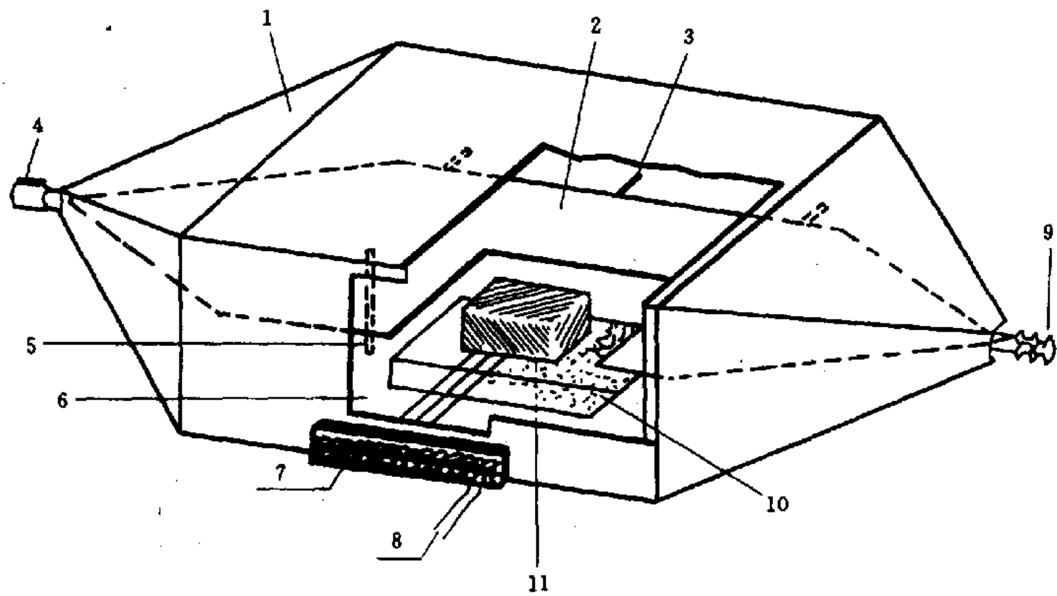
1—外导体,屏蔽;2—内导体(芯板);3—绝缘体;4—输入端;5—绝缘体;6—门 7—接线板;8—被测物体电源;9—端接电阻 50\Omega (匹配负载);10—绝缘支架 11—被测 ESA(最大高度为小室底板到芯板距离的 1/3 )
